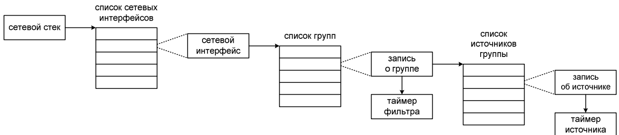
Фиг. 97. Структуры данных группового маршрутизатора — модель MLDv2
