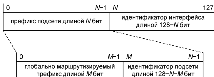
Фиг. 12. Общая структура глобального индивидуального адреса IPv6
