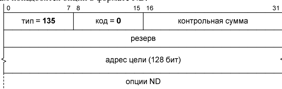
Фиг. 59. Вызов соседа — NS
