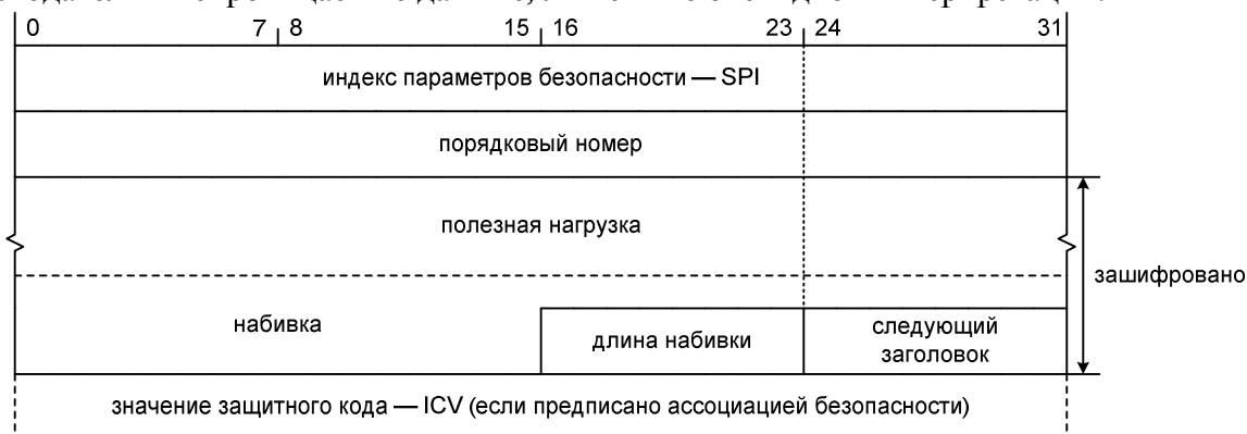
Фиг. 41. Инкапсуляция ESP
