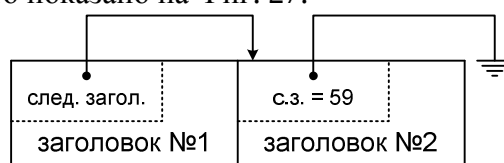
Фиг. 27. Пакет без полезной нагрузки
