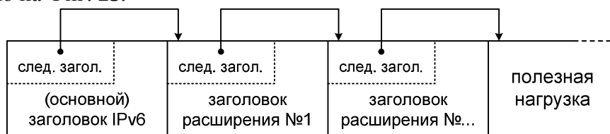
Фиг. 25. Окончательная структура пакета IPv6 (число заголовков расширения переменнo)
