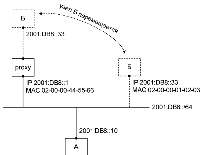
Фиг. 56. Мобильность узла, за которого отвечает ND proxy
