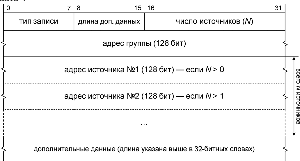
Фиг. 96. Запись о группе в отчете MLDv2
